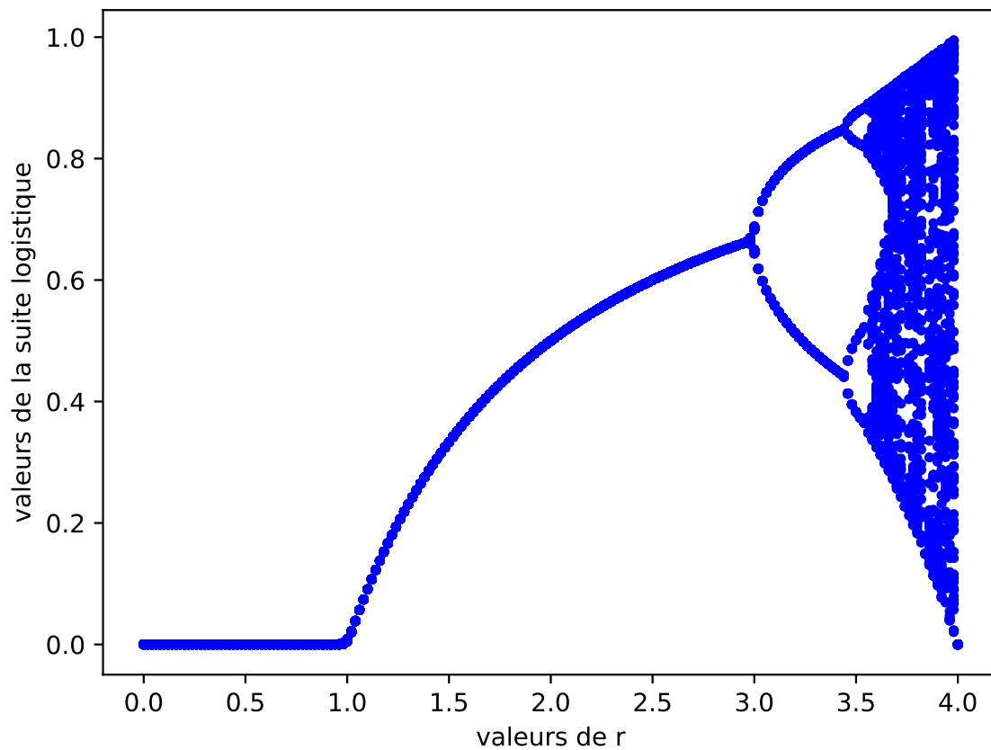
FIGURE 1 – Comportement de la suite logistique
